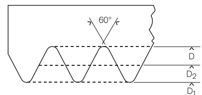
D 1 Kerndurchmesser D 2 Flankendurchmesser D Nennmaß des Gewindes/ Außendurchmesser
