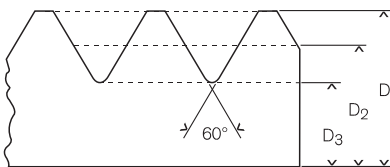
D 3 Kerndurchmesser D 2 Flankendurchmesser D Außendurchmesser
