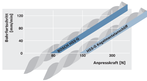
Metallbohrer HSS-G: bis zu 40 % schneller oder 50 % weniger Anpressdruck
