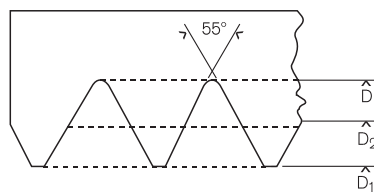
D 1 Kerndurchmesser D 2 Flankendurchmesser D Nennmaß des Gewindes/ Außendurchmesser
